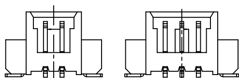
2 PIN 3 PIN LOCK CONFIGURATION 鎖扣位置
